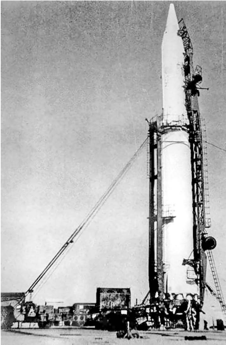
R-16 (8K64) – на пусковой установке
